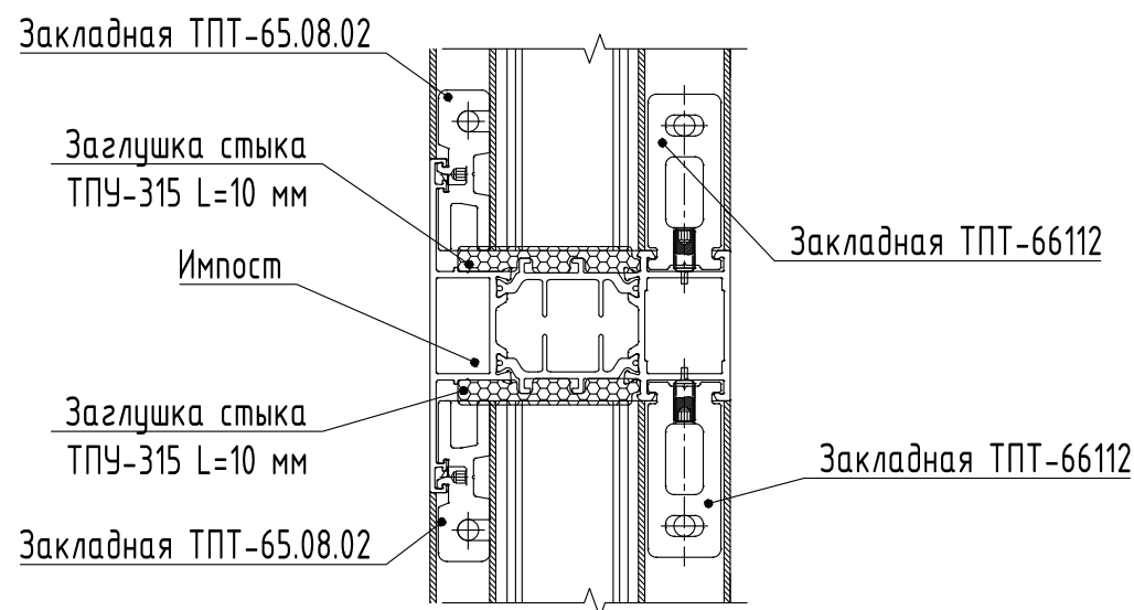
Заглушка стыка ТПУ-315
